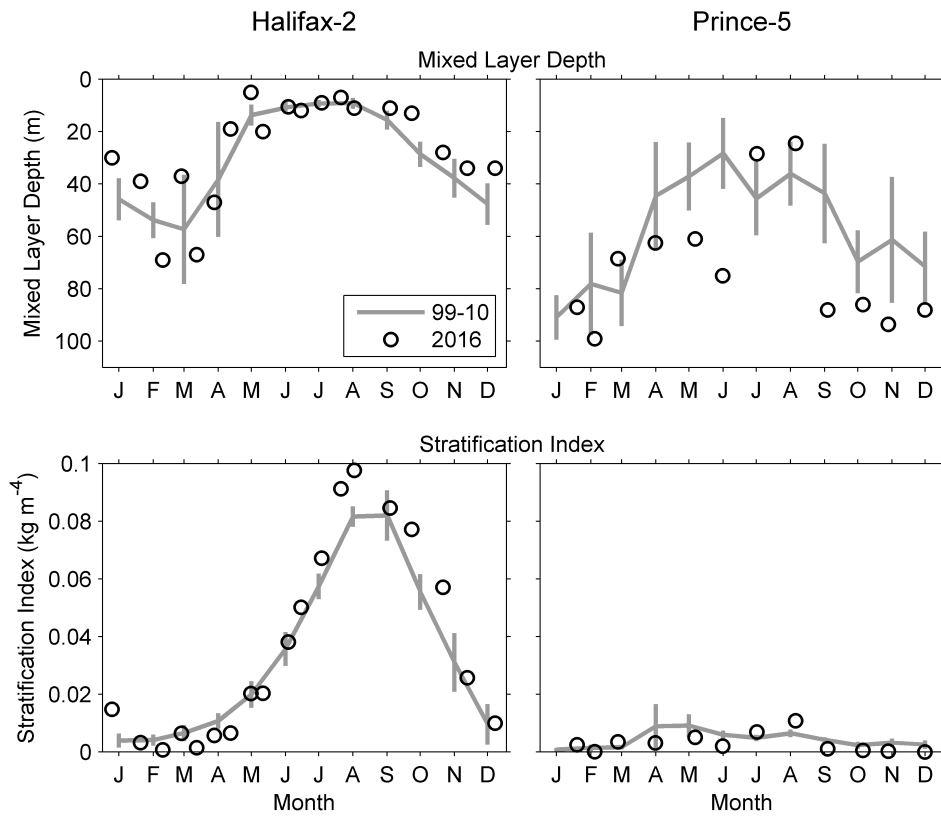
Propriétés de mélange (profondeur de la couche mélangée, indice de stratification) aux stations fixes des Maritimes comparant les données de 2016 (cercles) aux conditions moyennes de 1999-2010 (trait plein). Les lignes verticales sont les intervalles de confiance à 95% des moyennes mensuelles.
