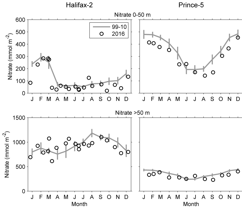
Variabilité annuelle de l'inventaire de chlorophylle aux stations fixes des Maritimes (Halifax-2 panneaux de gauche; Prince-5 panneaux de droite). Panneaux supérieurs: inventaire de chlorophylle (0-100 m pour Halifax-2, 0-95 m pour Prince-5) en 2015 (cercles) et valeurs moyennes de 1999-2010 (trait plein) . Les lignes verticales sont les intervalles de confiance à 95% des moyennes mensuelles. Panneaux du milieu: Cycle saisonnier moyen (1999–2010) de la structure verticale de la concentration de chlorophylle (mg m -3 ). Panneaux inférieurs: Cycle saisonnier de la structure verticale de la concentration de chlorophylle en 2015. L'échelle de couleur est choisie de manière à accentuer les changements correspondant approximativement aux niveaux de saturation alimentaire des gros copépodes.
