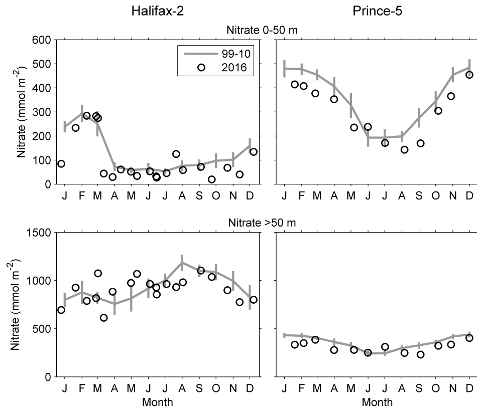
Comparaison des données de 2016 (cercles) aux conditions moyennes de 1999-2010 (trait plein) aux stations fixes des Maritimes. Panneaux supérieurs: inventaire de nitrate de surface (0-50 m). Panneaux inférieurs: inventaire de nitrate profond (>50 m). Les lignes verticales sont les intervalles de confiance à 95% des moyennes mensuelles.
